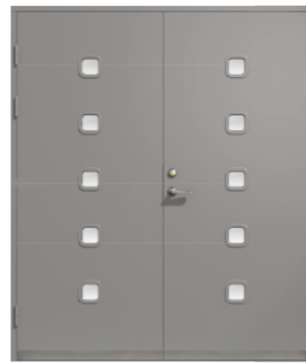
2YD 2001 Tjugohundra Pardörr visas här med dörrblad i lika bredd. Karmyttermått här M19x21.
