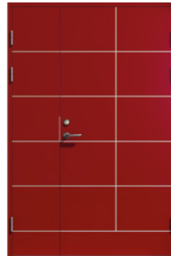
2YD 7 Kyoto Pardörr visas här med bredare gångdörr i modul 10. Karmyttermått här M15x21.
