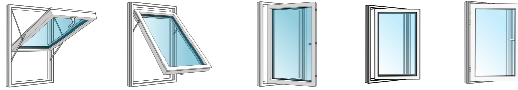
TSG 180 Horisontellt glidhängt 180° öppning TSG 45 Horisontellt glidhängt 45° öppning SSG 90 Vertikalt glidhängt 90° öppning SSG 180 Vertikalt glidhängt 180° öppning SHUG Sidohängt Öppnas utåt
