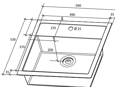
Håltagningsmått
