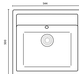
Håltagningsmått
