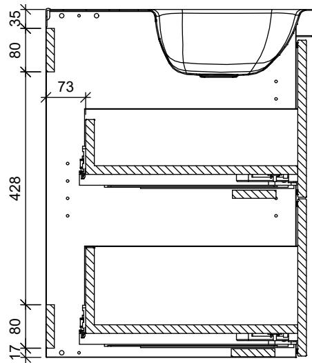
A-A
