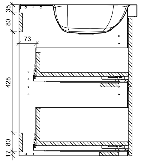
A-A
